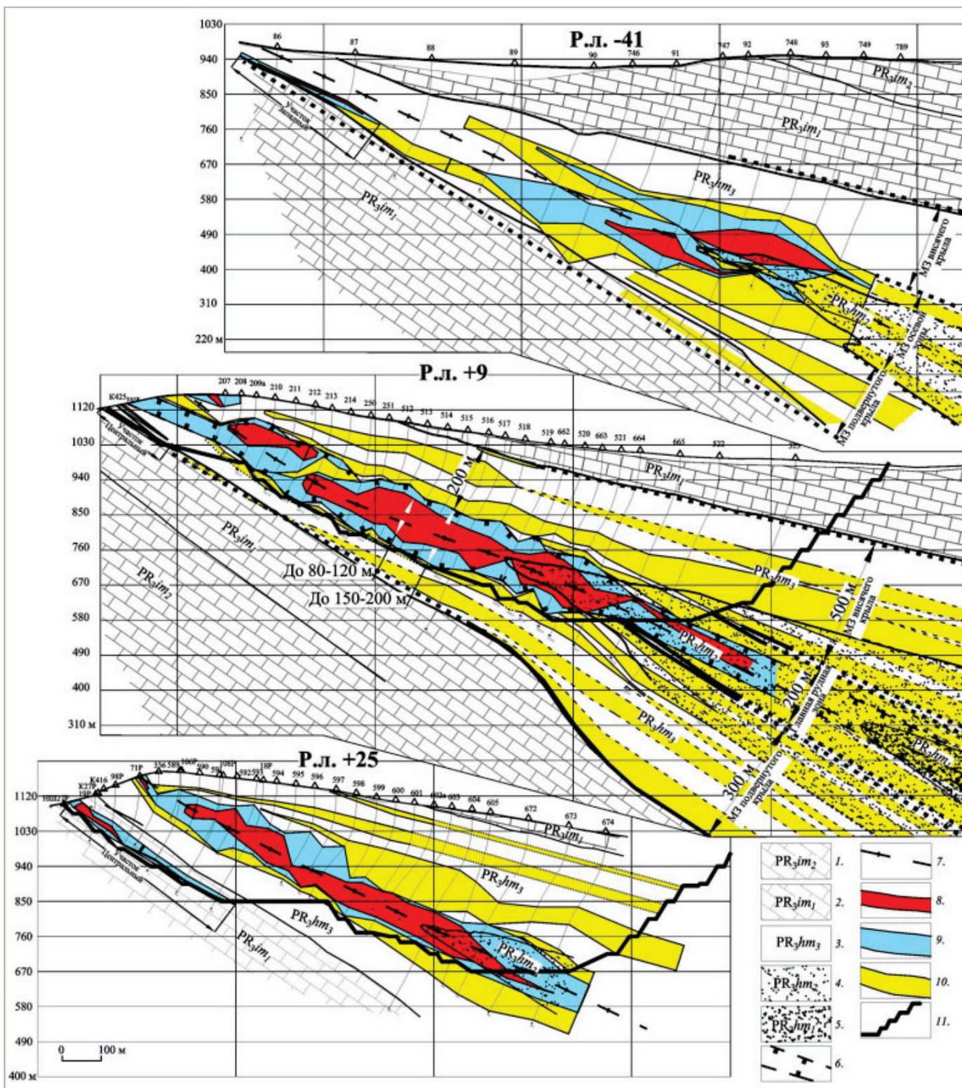
Рис. 3. Морфология и условия залегания рудных тел в разрезах по разведочным линиям: -41 (Северо-Западный и Западный участки), +9, +25 (Сухоложский и Центральный участки)
