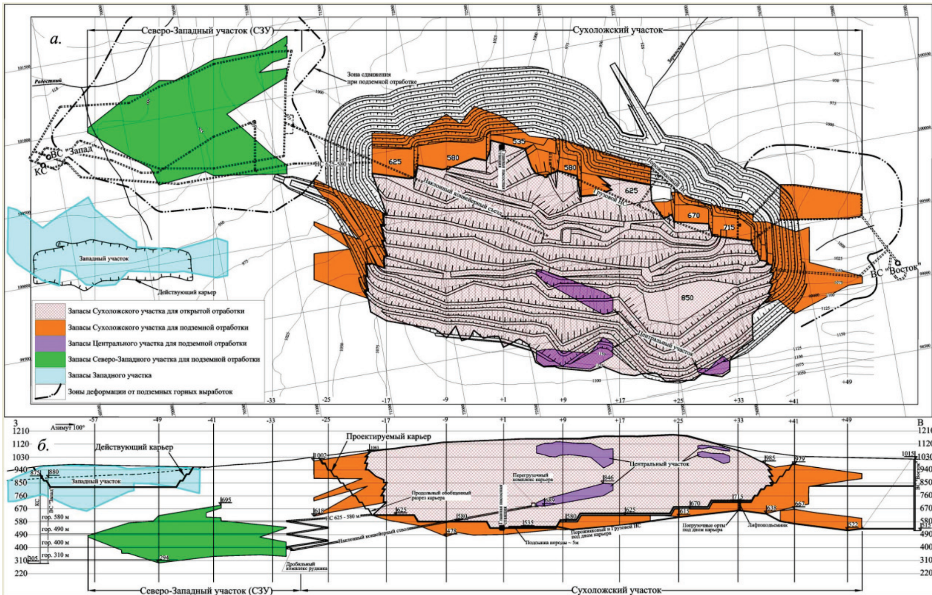
Рис. 5. Схема вскрытия месторождения в проекции на горизонтальную плоскость (а) и на продольную вертикальную плоскость (б)
